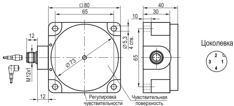
Габаритный чертёж
